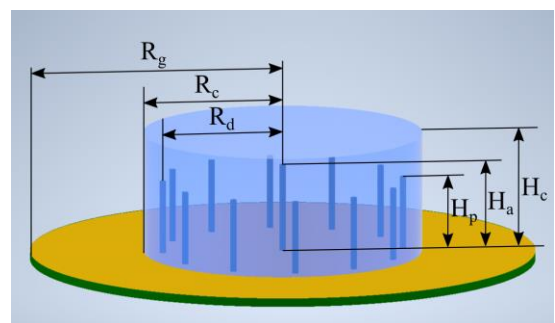
Fig. 1. Miniaturized ESPAR antenna structure
