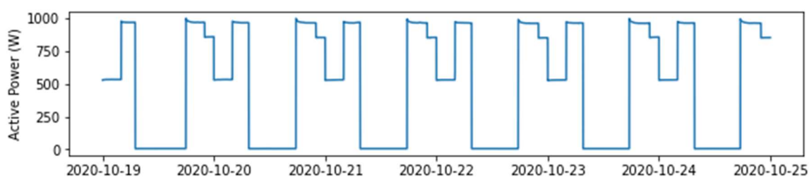
Rys. 4. Wykres mocy czynnej jednej fazy dla lamp z redukcją
