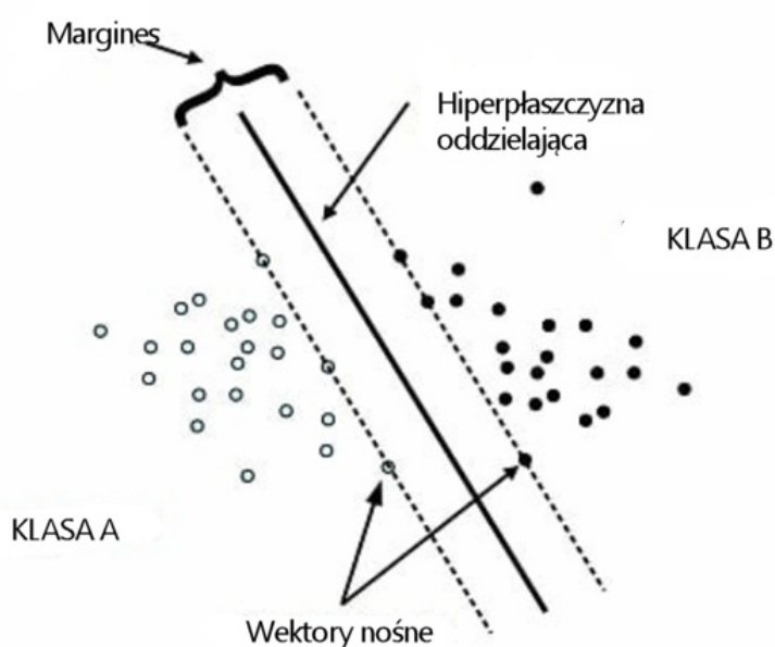
Rysunek 4.15: Ilustracja klasyfikatora SVM i miar go opisujących [129]
