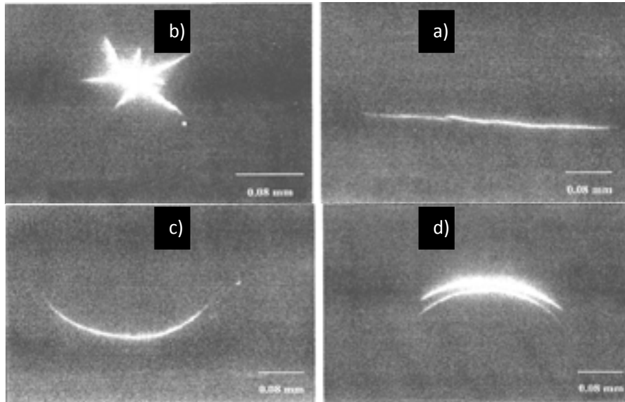
Rys. 1. Typowe wady spotykane na powierzchni kulek ceramicznych: a) pęknięcie gwiazdźdźiste, b) pęknięcie powstałe w wyniku procesu spiekania, c) pojedyncze pęknięcie kolistę, d) wielokrotne pęknięcie kolistę [L. 1]
