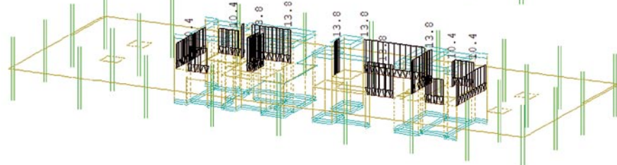
Rys. 10. Obciążenie od ścian murowanych – SOFiSTiK Wingraf
