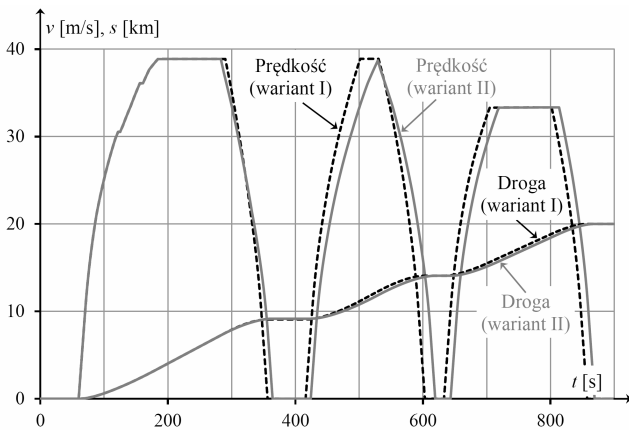
Rys. 6. Przebieg prędkości i położenia pojazdu
