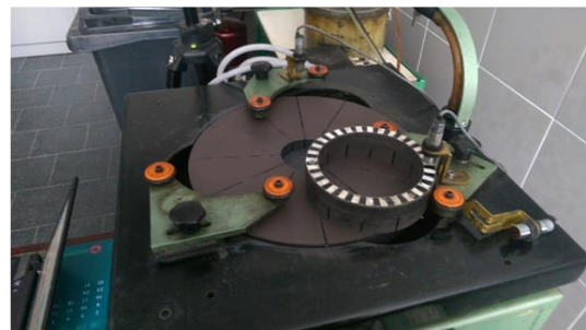
Rys.3. Widok układu wykonawczego docierarki jednotarczowej ABRALAP 380 (założony jeden pierścień prowadzący)
