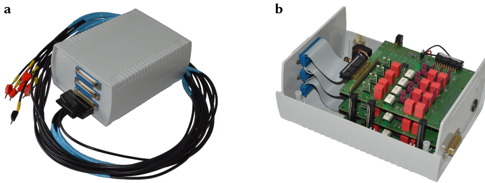
Rysunek 4.12. Urządzenie wykorzystane do powierzchniowego pomiaru aktywności bioelektrycznej mięśni podczas badań: a) widok z podłączonymi czterema sondami pomiarowymi; b) wnętrze urządzenia
