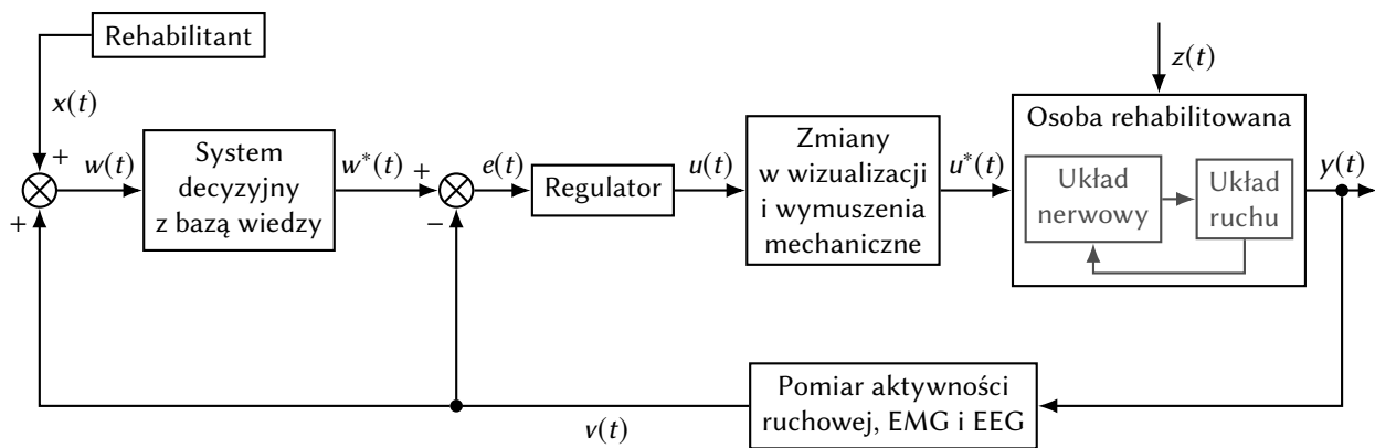
Rysunek 1.2. Schemat propozycji układu regulacji typu HITL do zastosowania w rehabilitacji
