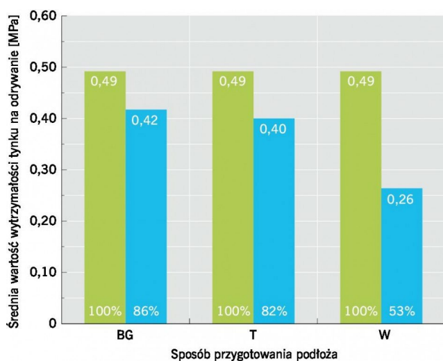
RYS. 6. Wykres średniej wytrzymałości na odrywanie tynku od podłoża (przyczepności) w funkcji sposobu jego przygotowania: tynk gipsowy na podłożu betonowym (ścianie żelbetowej). Oznaczenia próbek zgodnie z TABELĄ 1 (kolor zielony - wartość referencyjna); rys.: autorzy
