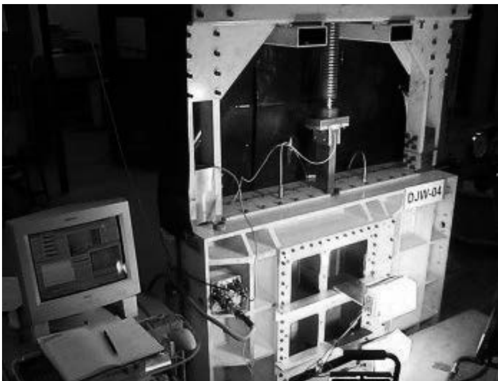
Рыс. 1. Комора калібрасьіейна в пласкїм станіе одксытасьлаленіа [30]
