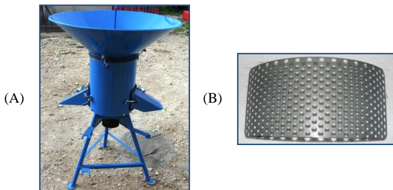
Rysunek 19. Rozdrabniacz rolniczy typu „Bąk” (A) oraz sitko o perforacji 8 mm (B)
