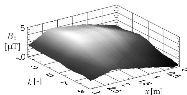
Rys.4. Przykładowy wykres rozkładu indukcji magnetycznej modelu okrętu; k – numery kolejne magnetometrów (wzdłuż osi y ), x – współrzędna wzdłuż osi x
