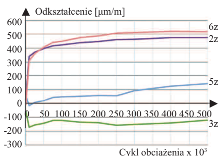
Rys. 6. Odkształcenia materiału GRP (zewnątrznej warstwy e_s ) profilu o grubości ścianki 35 mm w czasie badań pod obciążeniem zmiennym
