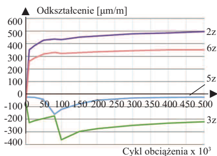
Rys. 5. Odkształcenia materiału GRP (zewnątrznej warstwy e_s ) profilu o grubości ścianki 45 mm w czasie badań pod obciążeniem zmiennym
