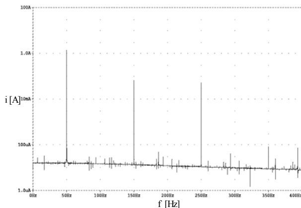
Rys. 2. Widmo prądu stojana, uzyskane w programie PSpice dla przypadku prostego obwodu RL z rezystancją stałą w czasie
