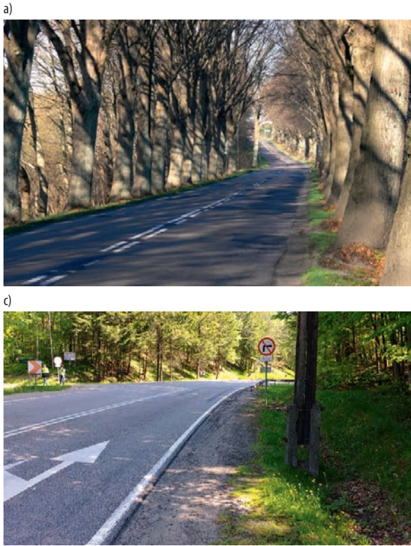
Rys. 3. Przykłady źródeł zagrożeń w otoczeniu drogi
