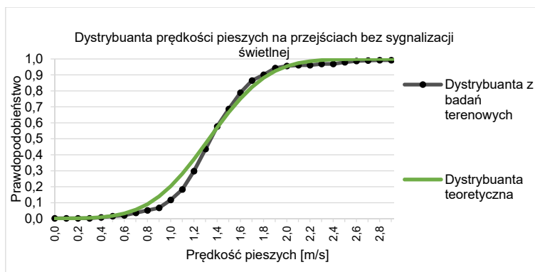
Rys.5.20 Dystrybuanta rozkładu prędkości pieszych na przejściu bez sygnalizacji świetlnej (dystrybuanta rzeczywista i teoretyczna dla rozkładu normalnego),
