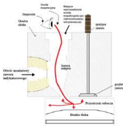
Rys. 5. Przekrój wzdłużny głowicy cylindrowej silnika "Farymann Diesel" typu D10 z zaznaczonym miejscem wprowadzenia sondy wziernikowej wideoendoskopu
