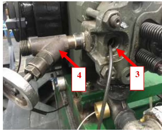
Rys. 4. Widok ogólny stanowiska laboratoryjnego silnika Farymann Diesel typu D10 przygotowanego do badań endoskopowych (a), sposób wprowadzenia sondy inspekcyjnej wideoendoskopu do przestrzeni roboczej silnika (b): 1 – silnik Farymann Diesel typu D10; 2 - wideoendoskop pomiarowy Everest typu XLG3 przygotowany do badania silnika; 3 – otwór wziernikowy po zdemontowanym wtryskiwaczu; 4 – zawór indykatorowy
