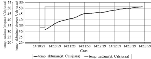
Rys. 4. Przebiegi temperatury mierzonej i zadanej przy wymuszeniu skokowym (grzanie) [4]
