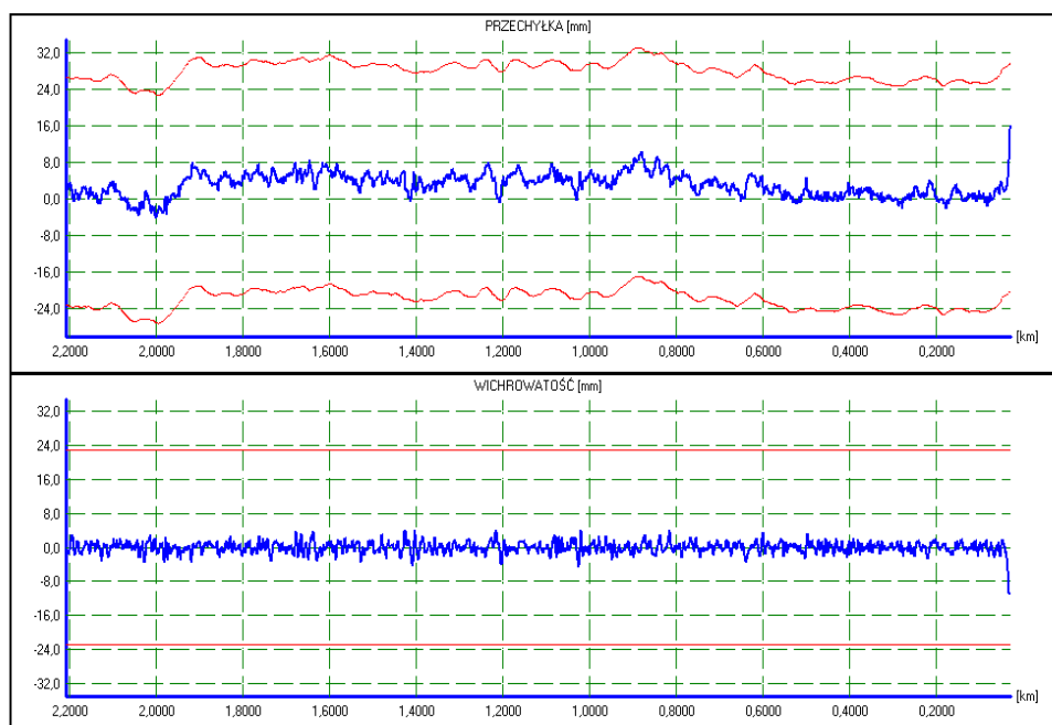
Rys. 3. Wykres przechyłki i wchrowatości toru
