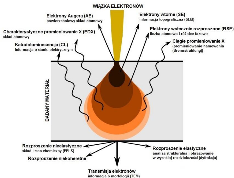
Rys. 38. Sygnały emitowane z różnych głębokości badanej próbki w wyniku oddziaływania z wysokoenergetyczną wiązką elektronów [607].
