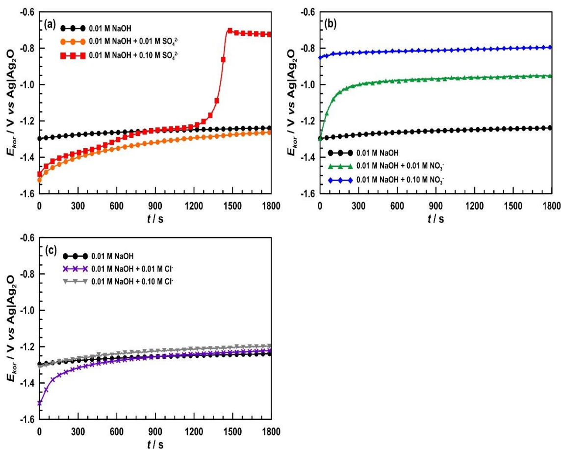
Rys. 83. Zmiany potencjału korozyjnego w funkcji czasu E_{kor} = f(t) zarejestrowane dla stopu aluminium AA2024 eksponowanego w 0.01 mol/dm 3 roztworze NaOH z dodatkiem jonów: (a) \text{SO}_4^{2-} , (b) \text{NO}_3^- , (c) \text{Cl}^- . Czas pomiaru: 1800 s.
