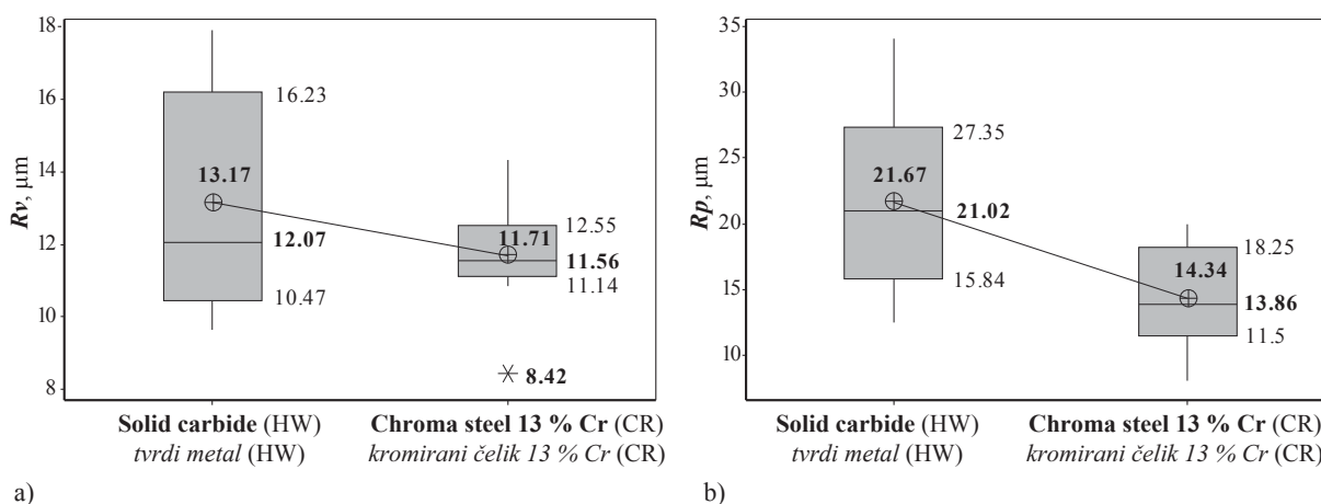
Figure 8 The mean value and value dispersion of maximum profile: valley depth R_v (a) and peak height R_p (b) vs. selected types of blade material (the box plot presents: the mean, median, interquartile range box and data range - outlier) Slika 8. Srednja vrijednost i rasipanje podataka: a) o dubini udoline R_v i b) o visini vrha R_p maksimalnog profila površine obrađene dvama različitim noževima (na grafu su prikazane srednje vrijednosti, medijani, interkvartilni raspon i raspon podataka)
