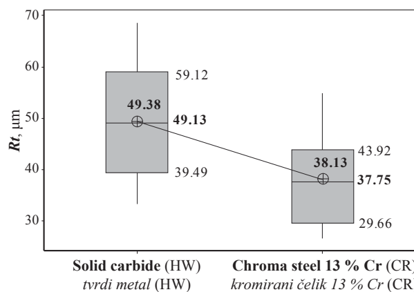
a) b) Figure 6 The mean value and value dispersion of total height Rt (a) and maximum height Rz (b) of the profile vs. selected types of blade material (the box plot presents: the mean, median, interquartile range box and data range) Slika 6. Srednja vrijednost i rasipanje podataka: a) o ukupnoj visini Rt i b) o maksimalnoj visini Rz profila obrađene površine pri obradi dvama različitim noževima (na grafu su prikazane srednje vrijednosti, medijani, interkvartilni raspon i raspon podataka)
