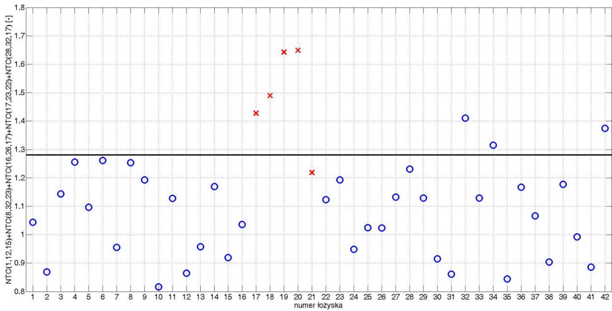
Rys. C. 35. Wartość wskaźnika diagnostycznego dla poszczególnych łożysk dla zestawu 1 bez obciążenia
