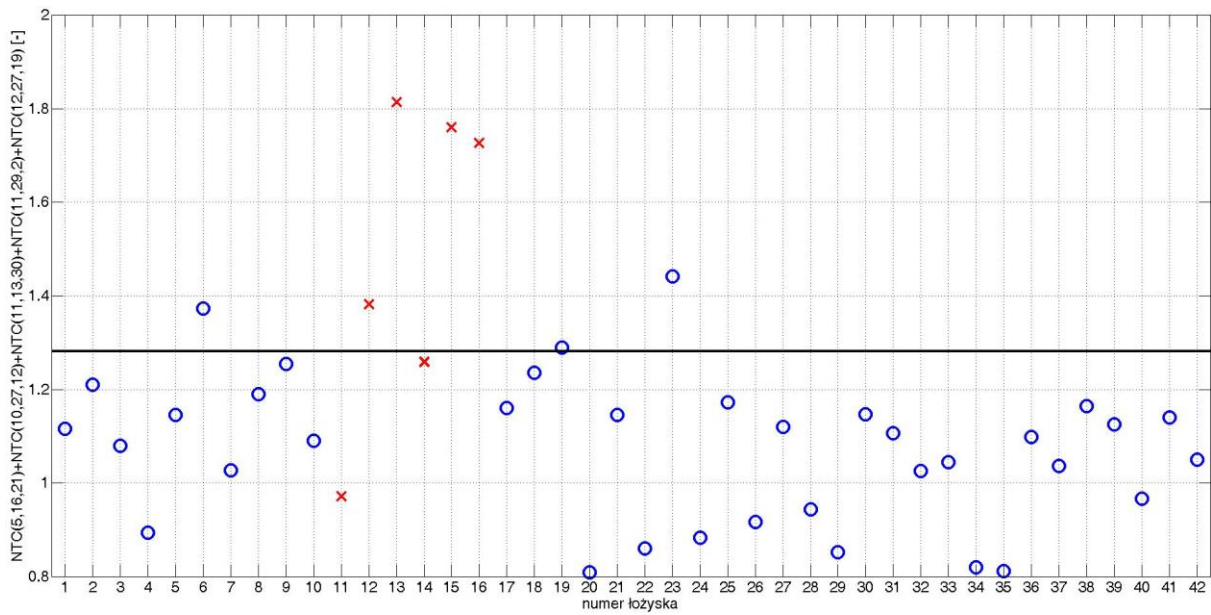
Rys. B. 3. Wartość wskaźnika diagnostycznego dla poszczególnych łożysk dla zestawu 4 przy obciążeniu 1,1 kW
