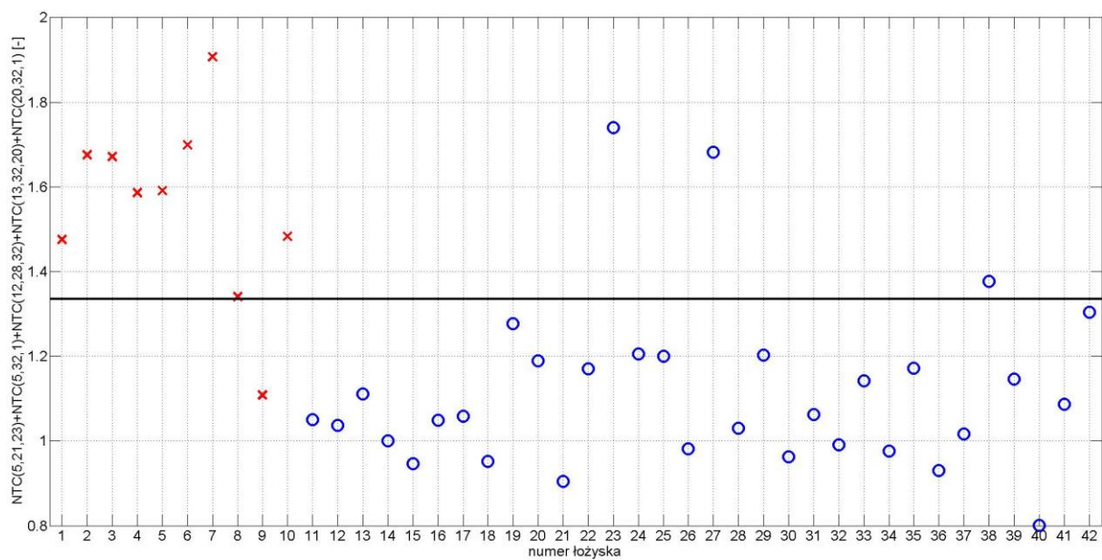
Rys. A. 10. Wartość wskaźnika diagnostycznego dla poszczególnych łożysk dla zestawu 1 przy obciążeniu 0,9 kW
