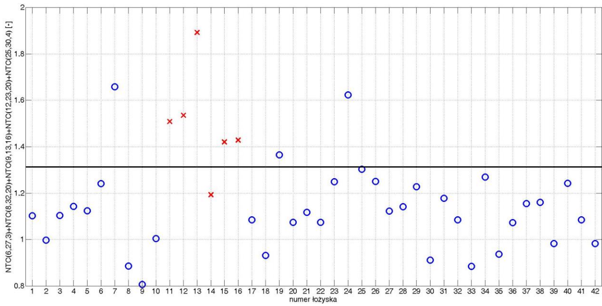
Rys. B. 11. Wartość wskaźnika diagnostycznego dla poszczególnych łożysk dla zestawu 2 przy obciążeniu 0,9 kW
