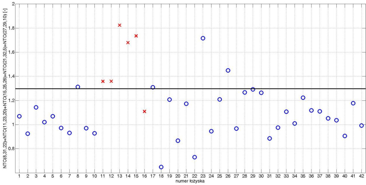
Rys. B. 7. Wartość wskaźnika diagnostycznego dla poszczególnych łożysk dla zestawu 3 przy obciążeniu 1,0 kW
