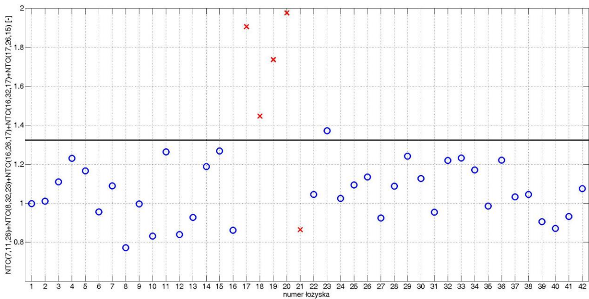
Rys. C. 36. Wartość wskaźnika diagnostycznego dla poszczególnych łożysk dla zestawu 2 bez obciążenia
