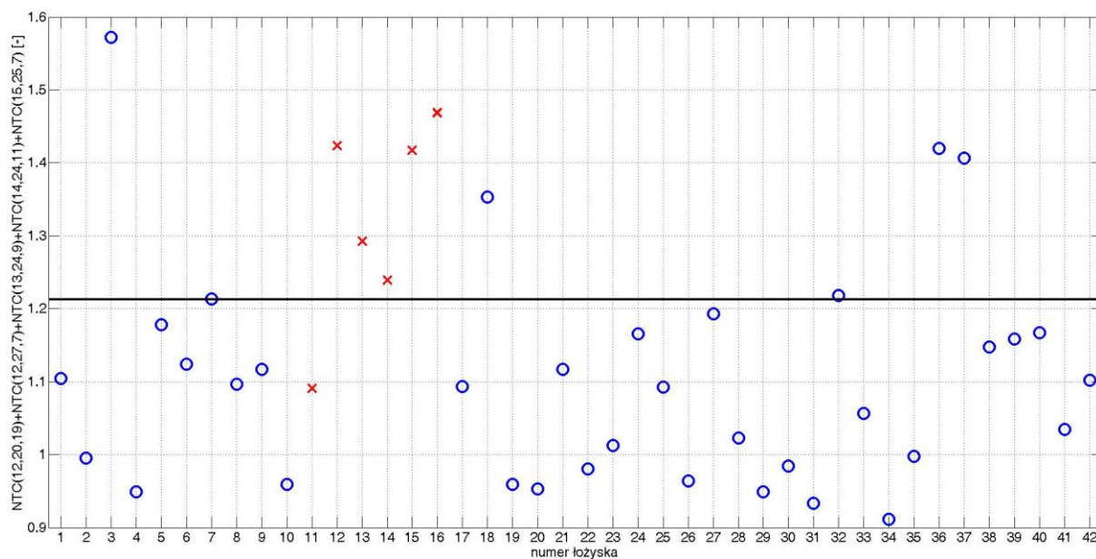
Rys. B. 2. Wartość wskaźnika diagnostycznego dla poszczególnych łożysk dla zestawu 3 przy obciążeniu 1,1 kW
