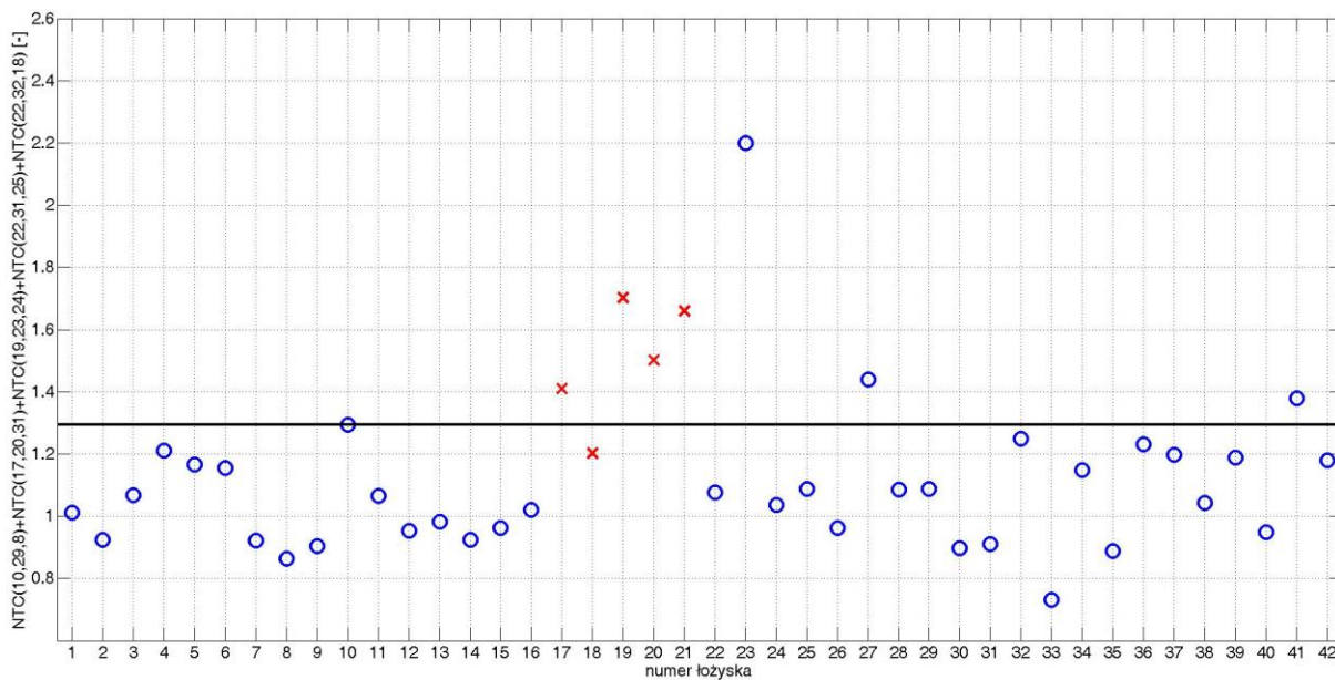
Rys. C. 5. Wartość wskaźnika diagnostycznego dla poszczególnych łożysk dla zestawu 1 przy obciążeniu 1,0 kW
