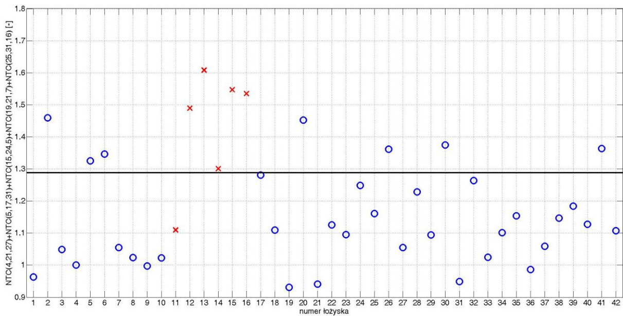
Rys. B. 16. Wartość wskaźnika diagnostycznego dla poszczególnych łożysk dla zestawu 2 przy obciążeniu 0,8 kW
