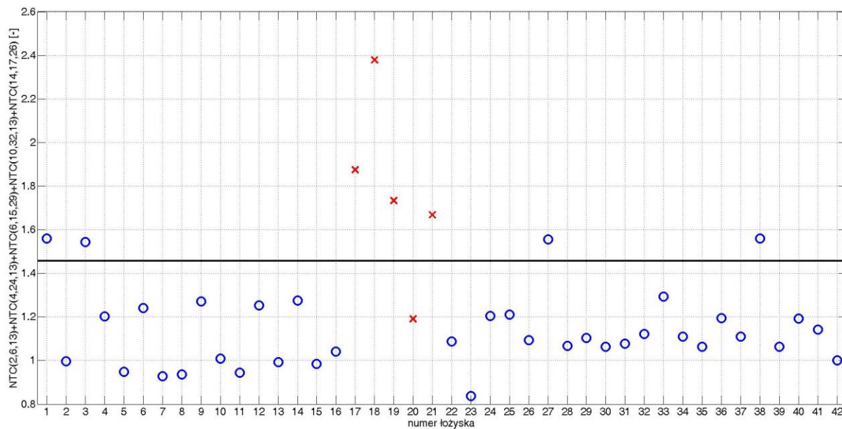
Rys. C. 3. Wartość wskaźnika diagnostycznego dla poszczególnych łożysk dla zestawu 4 przy obciążeniu 1,1 kW
