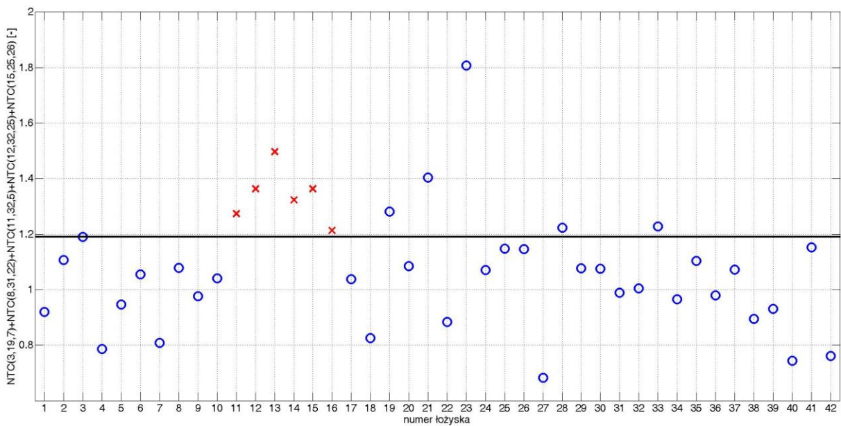
Rys. B. 8. Wartość wskaźnika diagnostycznego dla poszczególnych łożysk dla zestawu 4 przy obciążeniu 1,0 kW
