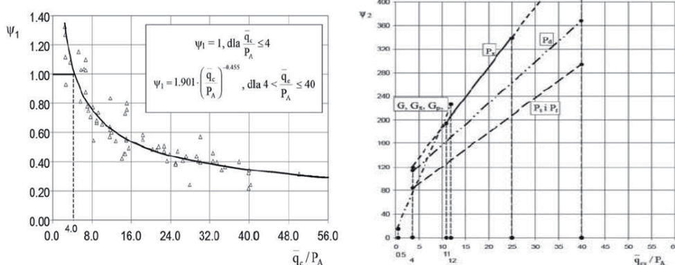
FIGURE 7. Capacity coefficients for Vibro piles in the Gwizdała–Stęczniewski method (Gwizdała, 2013)
