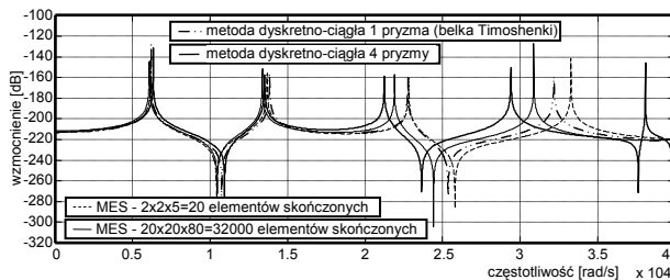
Rys. 5. Charakterystyki częstotliwościowe
