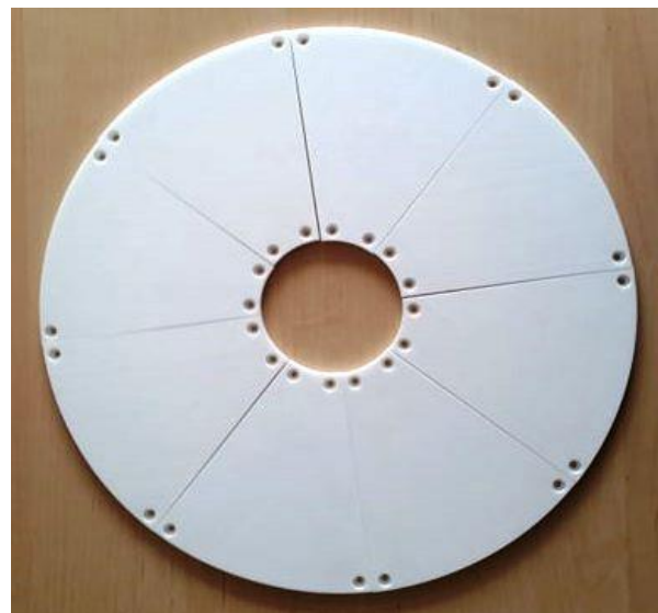
Rysunek 25. Prototypowa tarcza docierająca wykonana metodą SLS: a) widok pojedynczego segmentu ściernego; b) tarcza docierająca złożona z ośmiu segmentów ściernych
