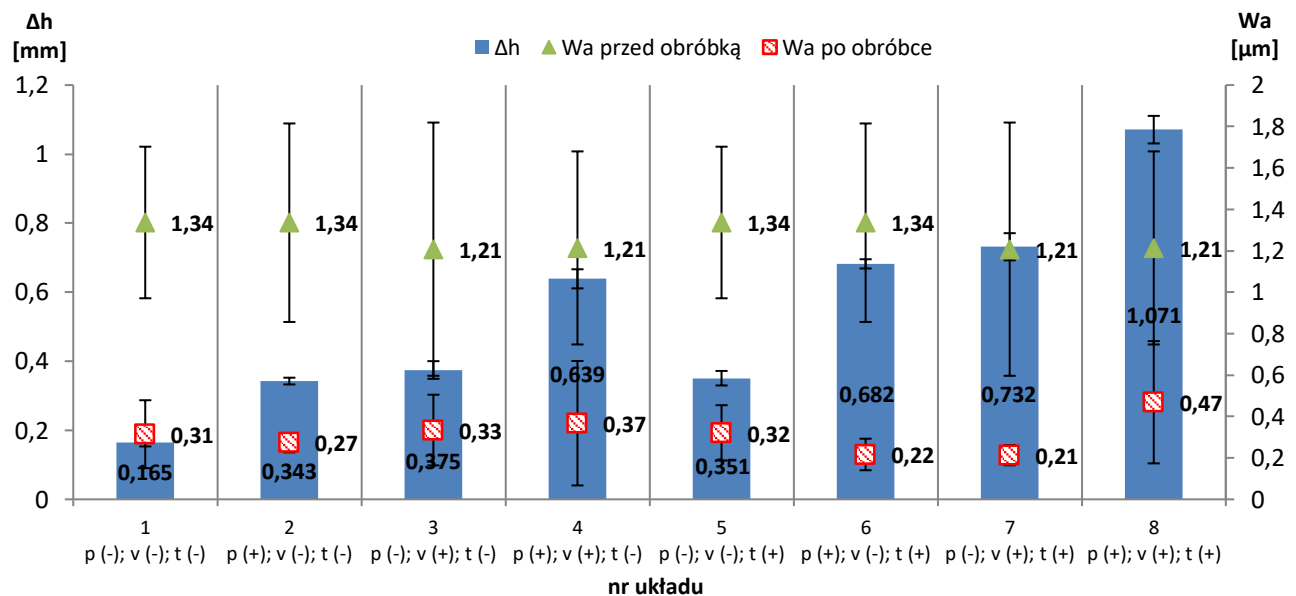
Rysunek 88. Efekty technologiczne uzyskane w poszczególnych układach badań eksperymentalnych docierania ceramiki technicznej: a) masowy ubytek materiałowy \Delta m oraz chropowatość powierzchni Ra; b) liniowy ubytek materiałowy \Delta h oraz falistość powierzchni Wa
