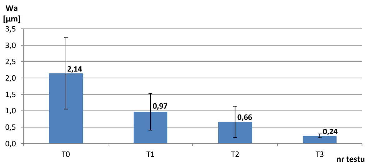
Rysunek 48. Wartości parametrów chropowatości oraz falistości po określonych testach docierania jednostronnego próbek z ceramiki technicznej \text{Al}_2\text{O}_3 (T0 – stan początkowy próbek przed rozpoczęciem obróbki):
