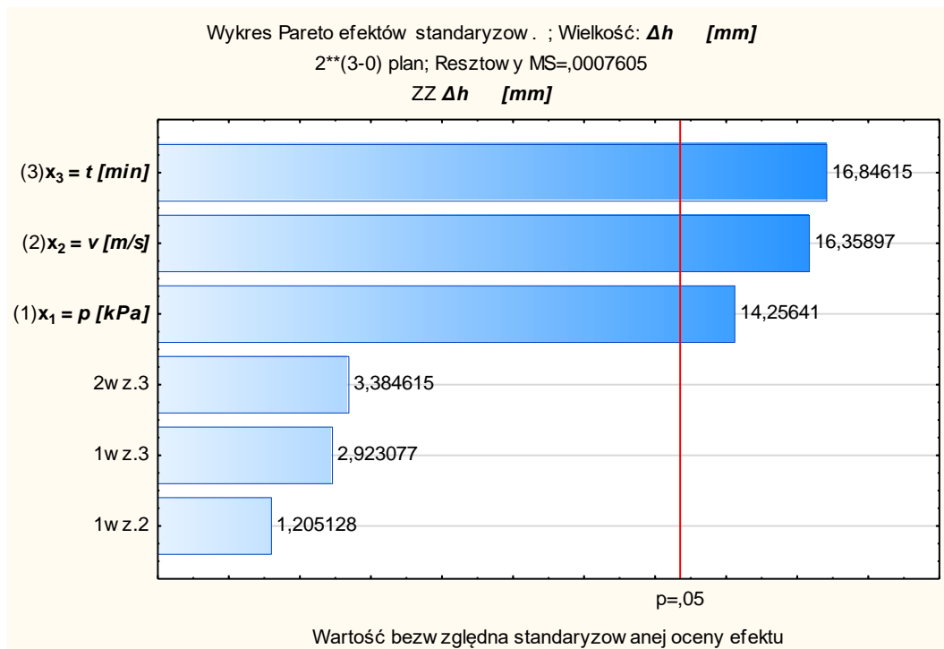
Rysunek 93. Wykresy Pareto efektów standaryzowanych wielkości wejściowych i ich interakcji dla ubytku materiałowego: a) masowego \Delta m ; b) liniowego \Delta h
