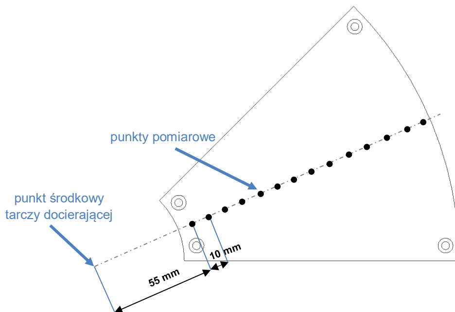
Rysunek 44. Miejsca wykonywanych pomiarów dla pojedynczego segmentu
