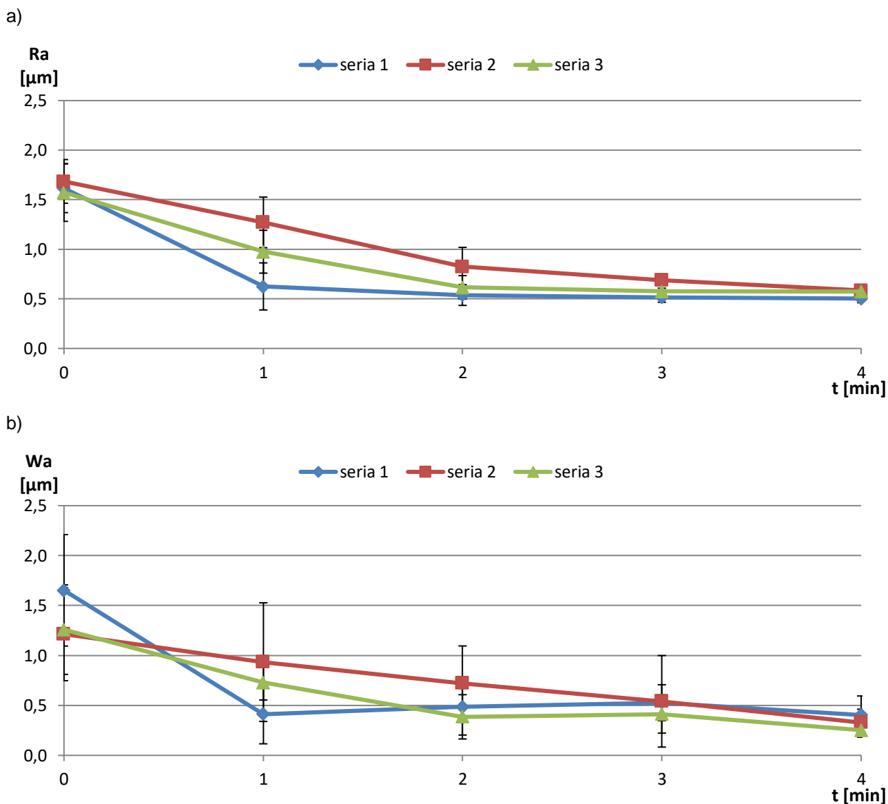
Rysunek 80. Wartości parametrów chropowatości Ra (a) i falistości Wa (b) uzyskane podczas badań sprawdzających docierania jednostronnego ceramiki technicznej Al_2O_3
