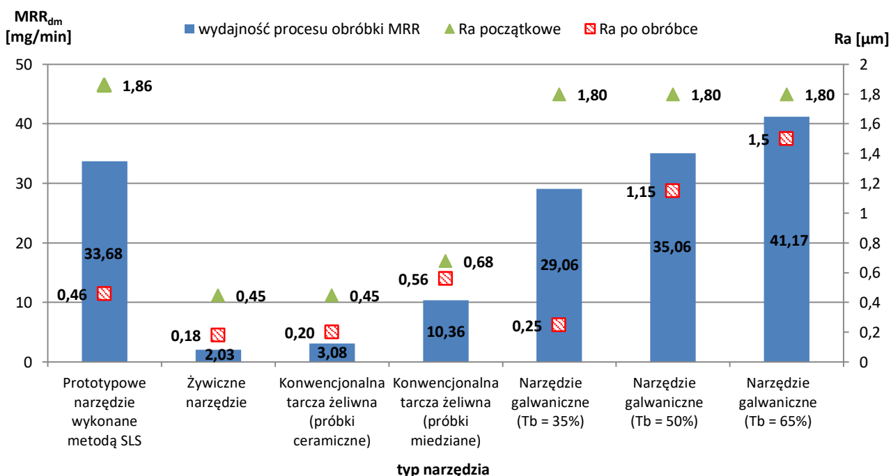
Rysunek 106. Porównanie wydajności procesu obróbki MRR_{dm} oraz parametru chropowatości R_a dla różnych typów narzędzi ściernych; kolejność zgodna z danymi w tabelach 25 oraz 26
