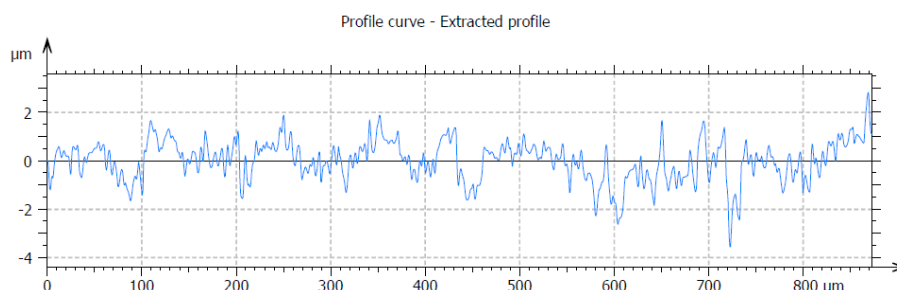
Rysunek 55. Trójwymiarowa analiza struktury powierzchni ceramiki technicznej po procesie docierania (zakończeniu badań rozpoznawczych): a) topografia powierzchni z wybranymi parametrami wysokościowymi; b) wyodrębniony profil powierzchni
