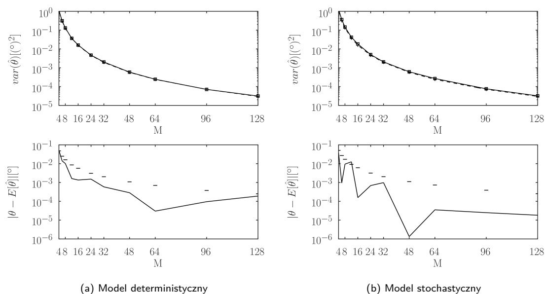
Rys. 7.29: Porównanie wariancji estymowanego kąta (linia ciągła, symbole kwadratu) z ograniczeniem Craméra-Rao (linia przerywana, symbole "+") w zależności od liczby elementów antenowych, dla danych wygenerowanych na podstawie modelu deterministycznego (7.29a) i stochastycznego (7.29b) wraz z wartością obciążenia (poziome kreski oznaczają górną granicę 95% przedziału ufności).
