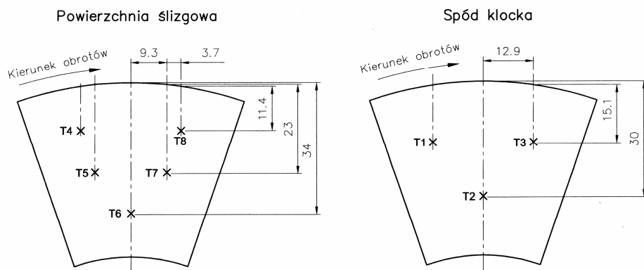
Rys. 4. Schemat rozmieszczenia termopar w klocku badawczym
