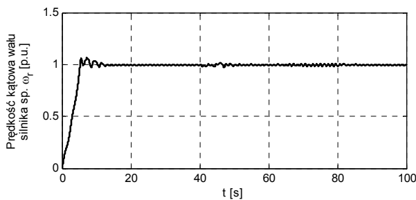
Rys. 6. Symulowany przebieg prędkości kątowej wału \omega_r silnika spalinowego. Oś rzędnych wyrażona w wartościach względnych, oś odciętych w sekundach
