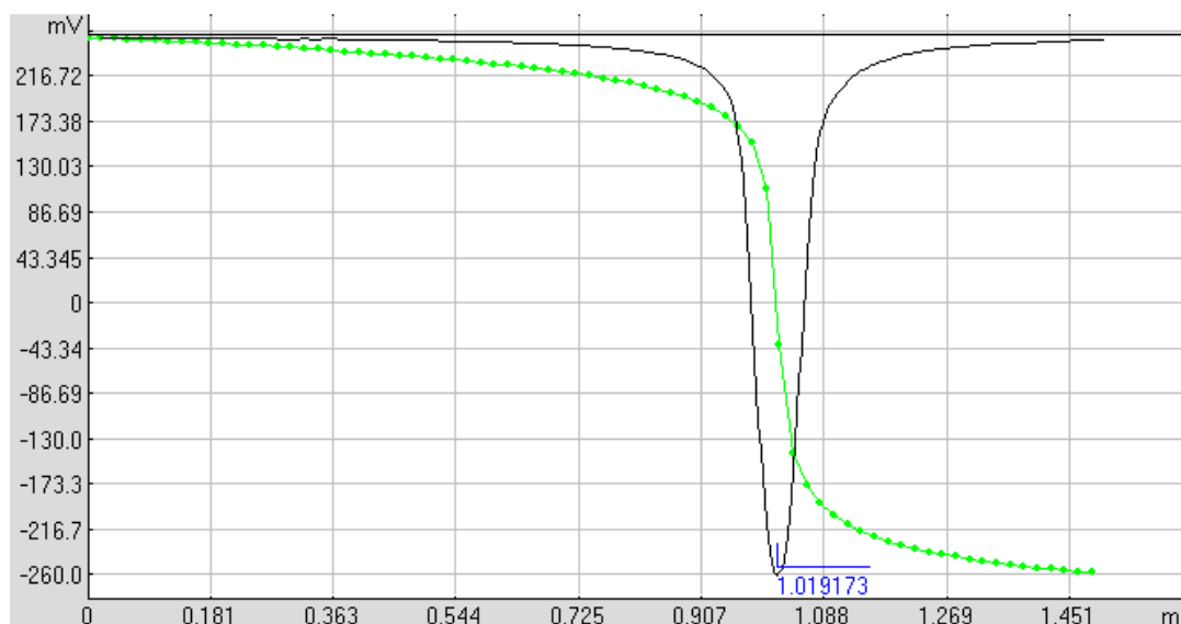
Rys. 64. Wyznaczanie miana roztworu HNO 3 . Zależność SEM(V NaOH ) oraz jej pochodna.
