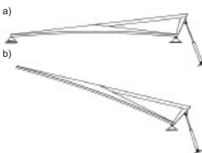
Rys. 1. Schemat kładki wraz z silownikiem: a) w pozycji opuszczonej; b) w pozycji otwartej
