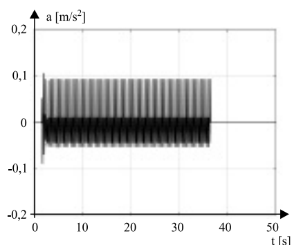
Rys. 4. Analiza numeryczna – składowa pionowa przyspieszenia konstrukcji przęsła w 1/2 rozpiętości – marsz swobodny 20-osobowej grupy [4]
