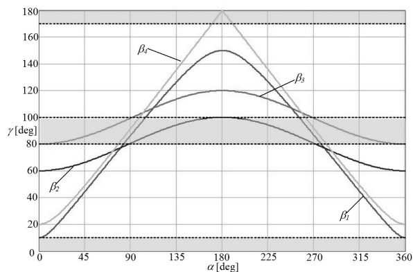
Rys. 6. Zależność kąta \gamma magnetometru w obszarze o inklinacji magnetycznej I = 10^\circ dla wybranych wartości kąta \beta ( \beta_1 = 110^\circ, \beta_2 = 160^\circ, \beta_3 = 20^\circ, \beta_4 = 80^\circ ) Fig. 6. The dependence of \gamma angle in the area of magnetic inclination I = 10^\circ for selected values of \beta angle ( \beta_1 = 110^\circ, \beta_2 = 160^\circ, \beta_3 = 20^\circ, \beta_4 = 80^\circ )
