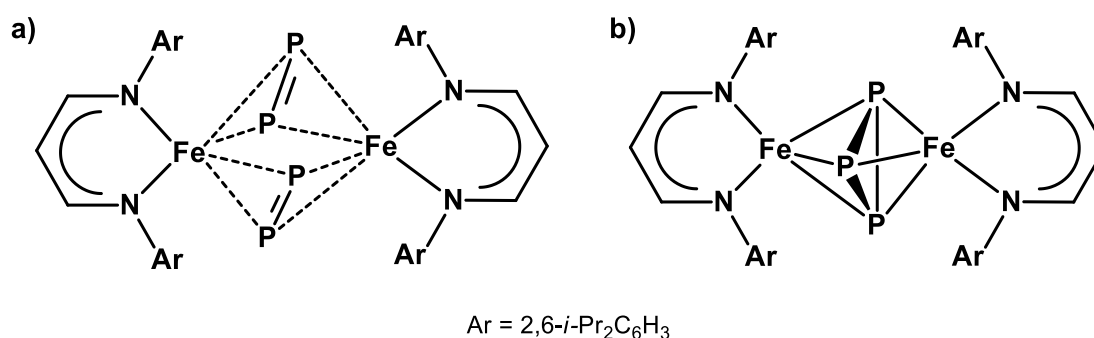
Rysunek 16. Przykłady kompleksów \beta -diketiminowych żelaza zawierających w swoich strukturach atomy fosforu: a) kompleks Fe(III) otrzymany w grupie badawczej Scheera 111 , b) kompleks Fe(II)Fe(III) otrzymany w grupie badawczej Driessa 15 .
