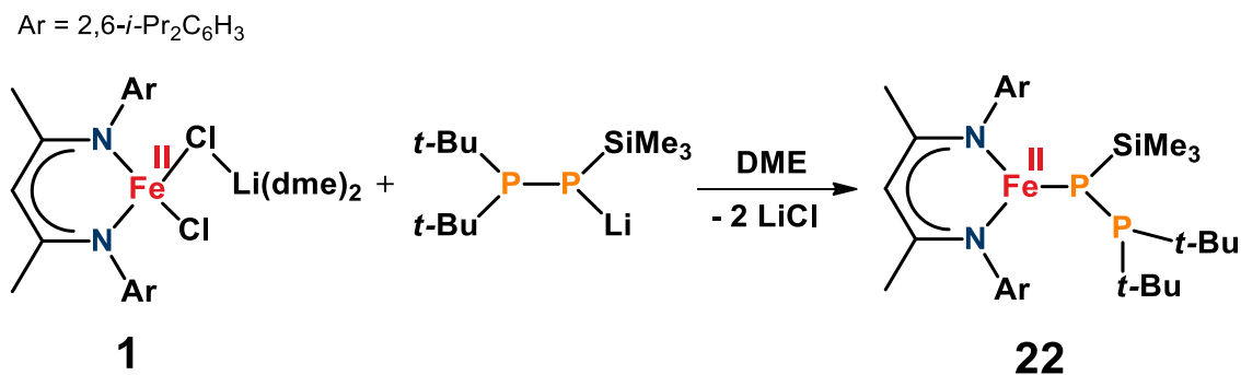
Rysunek 85. Reakcja syntezy terminalnego fosfanylofosfidowego kompleksu żelaza(II) [(Dippnacnac)Fe( \eta^1 -Me 3 SiPP- t\text{-Bu}_2 )] ( 22 ).
