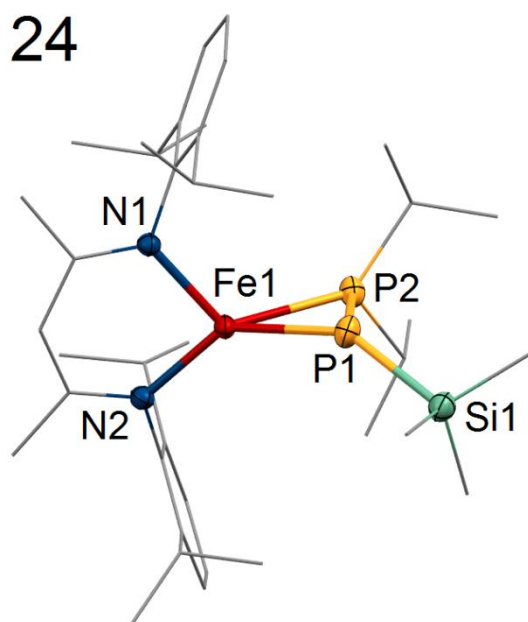
Rysunek 91. Struktura krystalograficzna terminalnego fosfanylofosfidowego kompleksu żelaza(II) [(Dippnacnac)Fe( \eta^2 - i -Pr 2 PPSiMe 3 )] (24). Dla lepszej czytelności rysunku atomy wodoru zostały pominięte. Elipsoidy termiczne 50%. Najważniejsze długości wiązań [Å] i kąty [°]: Fe1-N1 2,003(2); Fe1-N2 2,0218(19); Fe1-P1 2,3638(9); Fe1-P2 2,5070(10); P1-P2 2,1490(10); N1-Fe1-N2 93,02(8); P1-Fe1-P2 52,26(3); Fe1-P1-P2 67.30(4).
