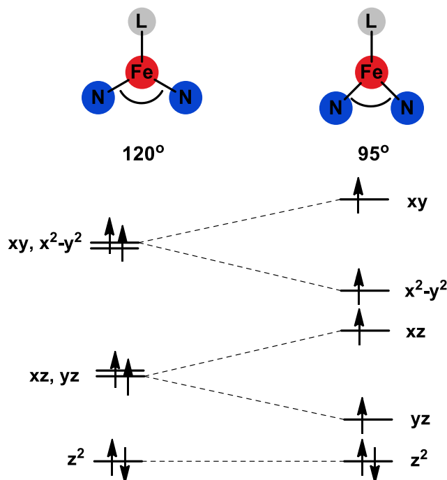
Rysunek 13. Zmiany w energii orbitali d spowodowane zniekształceniem geometrii w trójkordynacyjnym kompleksie z ligandem \beta -diketiminowym.
