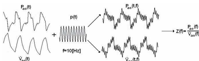
Rys. 2. Zasada pomiaru impedancji oddechowej z wykorzystaniem fali ciśnieniowej
