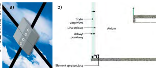
Rys. 8. Przykłady rozwiązań konstrukcyjnych ścian z oszkleniem mocowanym punktowo
