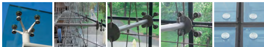
Rys. 8. Przykłady rozwiązań konstrukcyjnych ścian z oszkleniem mocowanym punktowo
