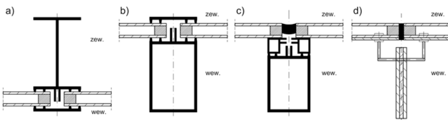
Rys. 5. Proces modyfikacji konstrukcji ściany słupowo-ryglowej a) Detal ściany słupowo-ryglowej starego typu. Konstrukcja ściany usytuowana na zewnątrz budynku, po jej stronie zimnej. Oszklenie ściany montowane od wewnątrz budynku b) Detal ściany słupowo-ryglowej nowej generacji. Konstrukcja ściany usytuowana na wewnętrznej stronie przegrody, po jej stronie ciepłej. Oszklenie ściany montowane od zewnętrznej strony budynku c) Detal ściany słupowo-ryglowej z oszkleniem strukturalnym. Konstrukcja ściany usytuowana po wewnętrznej stronie przegrody, po jej cieplej stronie. Oszklenie ściany montowane od strony zewnętrznej budynku d) Detal ściany osłonowej z punktowym (mechanicznym) mocowaniem oszklenia (nowej generacji). Konstrukcja przegrody usytuowana po jej stronie wewnętrznej (żebro szklane)
