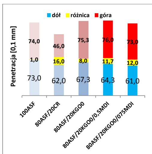
Rysunek 60 Stabilność w odniesieniu do penetracji dla asfaltów modyfikowanych za pomocą 20% mas. KGO0 oraz 0,50-0,75% mas. ciepłego MDI
