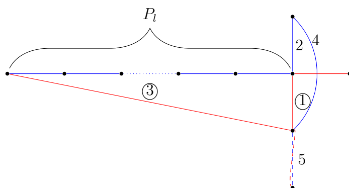
Rysunek 3.14: Kolejne tury gry dla podprzypadku 2.2 lematu 3.2.8.
