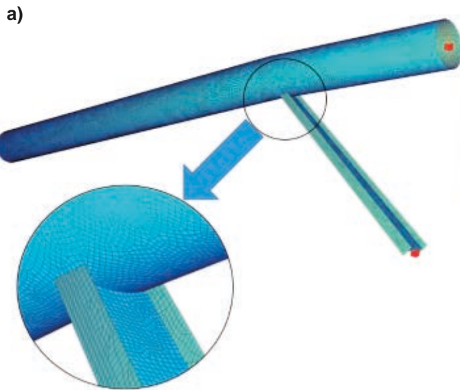
Rys. 7. Wizualizacja modelu obliczeniowego (W14) wersja pierwotna a) widok ogólny i szczegółowy modelu, b) sztywne elementy belkowe łączące krawędzie elementów powłokowych z punktem brzegowym
