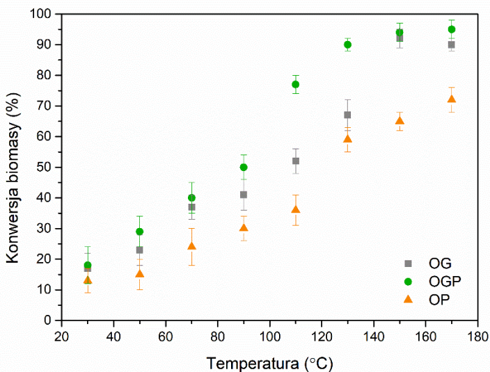
Rysunek 19. Zależność konwersji biomasy od temperatury w trakcie procesu upłynniania.
