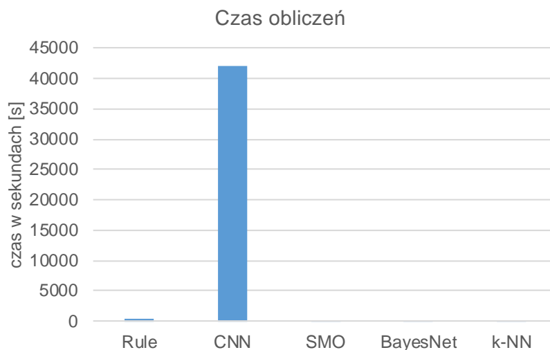
Rule CNN SMO BayesNet k-NN czas [s] 297 42213 15 35 11 Rysunek 5-13 Czas klasyfikacji dla poszczególnych algorytmów
