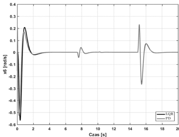
Rys. 2. Przebiegi prędkości kątowej drugiego ramienia wahadła
