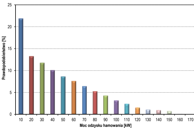
Rys. 4. Histogram mocy generowanej przez trolejbus podczas hamowania
