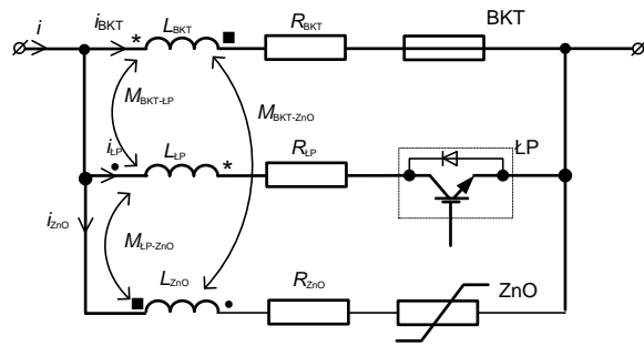
Rys. 3. Schemat zastępczy CHCL: L BKT – indukcyjność gałęzi BKT, L LP – indukcyjność gałęzi ŁP, L ZnO – indukcyjność gałęzi ZnO, R BKT – rezystancja własna gałęzi BKT, R LP – rezystancja gałęzi ŁP, R ZnO – rezystancja gałęzi ZnO, M BKT-LP – indukcyjność wzajemna gałęzi BKT i ŁP, M LP-ZnO – indukcyjność wzajemna gałęzi ŁP i ZnO, M BKT-ZnO – indukcyjność wzajemna gałęzi BKT i ZnO, i – prąd obwodu
