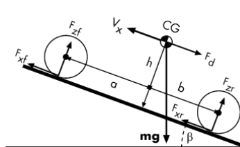
Rys. 2. Rozkład sił dla pojazdu na równi pochyłej [5]
