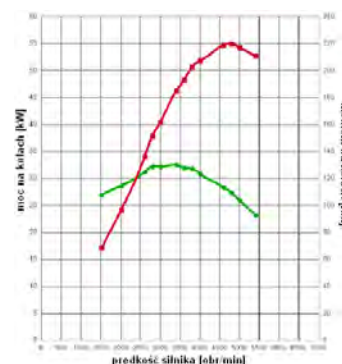
Rys. 3. Charakterystyka statyczna silnika [8]
