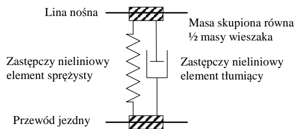
Rys. 4. Model wieszaka
