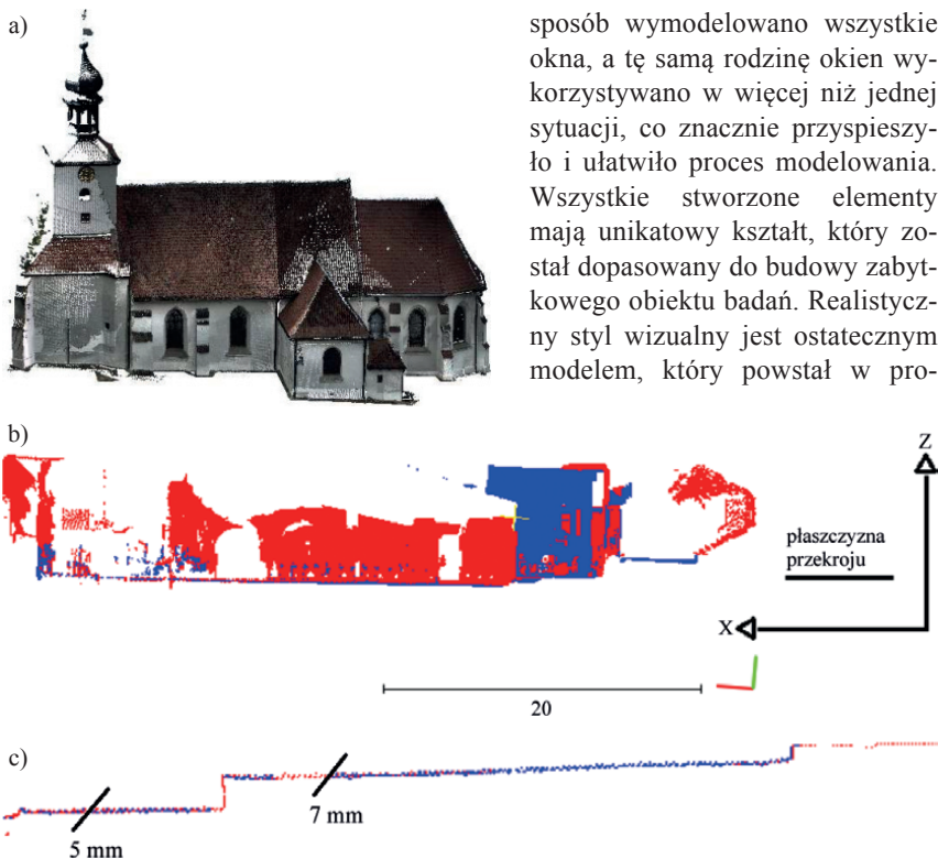
Rys. 1. Wynikowa chmura punktów: a) przekrój przez wynikową chmurę punktów; b) określenie maksymalnej odległości pomiędzy poszczególnymi skanami; c) precyzyjność łączenia skanów pokazana w przekroju
