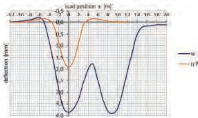
8. Zmiana ugięcia i linia wpływu ugięcia klucza powłoki
