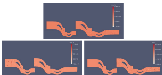
Rys. 4. Rozkład błędów względnego w neuralgicznym przekroju kanału przepływowego dla liczby Macha, ciśnienia oraz temperatury
