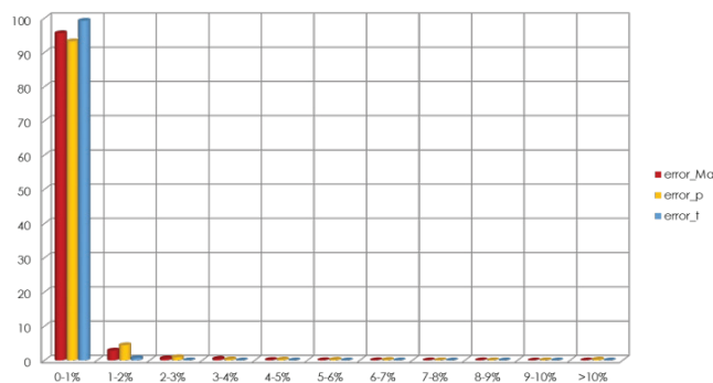
Rys. 5. Histogram przedstawiający liczebność wartości błędów względnych w poszczególnych przedziałach procentowych dla liczby Macha, ciśnienia oraz temperatury
