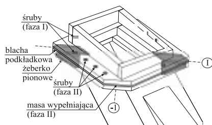
Rys. 6. Modyfikacja oparcia dźwigara na gałęzi słupa SD.II-2.1 (opis w tekście)
