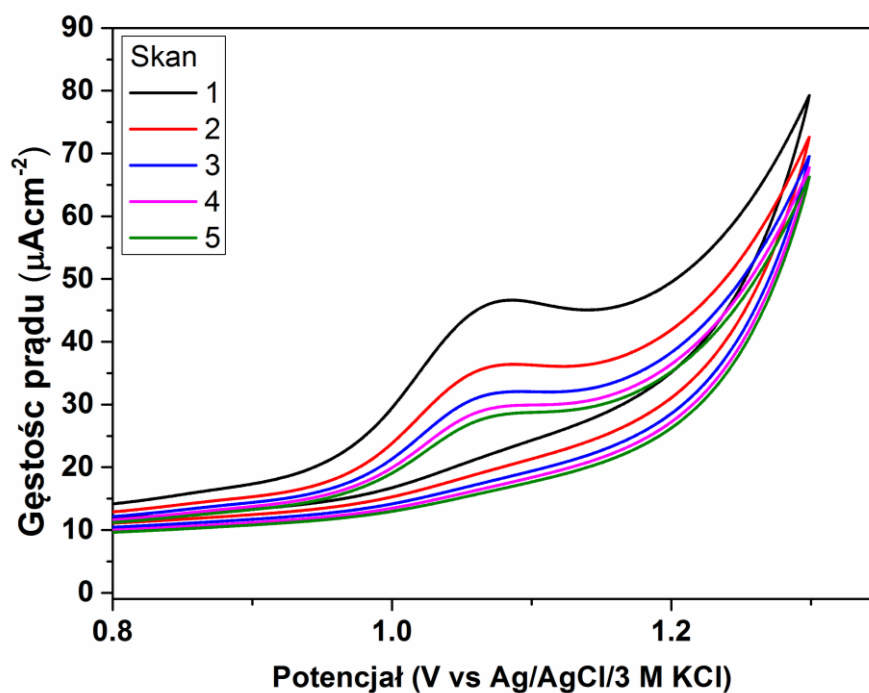
Rys. 47 Krzywe i-E pięciu następujących po sobie skanów dla roztworu isatinu 500 \mu\text{M} w 0,1 M pH = 7,2 PB.
