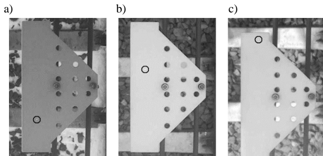
Rys. 5. Miejsce padania promienia lasera na płytkę refleksyjną przy temperaturze otoczenia: a) -14^{\circ}\text{C} , b) +12^{\circ}\text{C} , c) +30^{\circ}\text{C}
