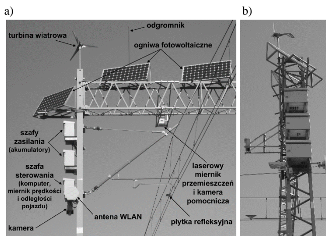
Rys. 4. Stanowisko pomiarowe na linii kolejowej: a) widok wzdłuż osi toru, b) widok z boku
